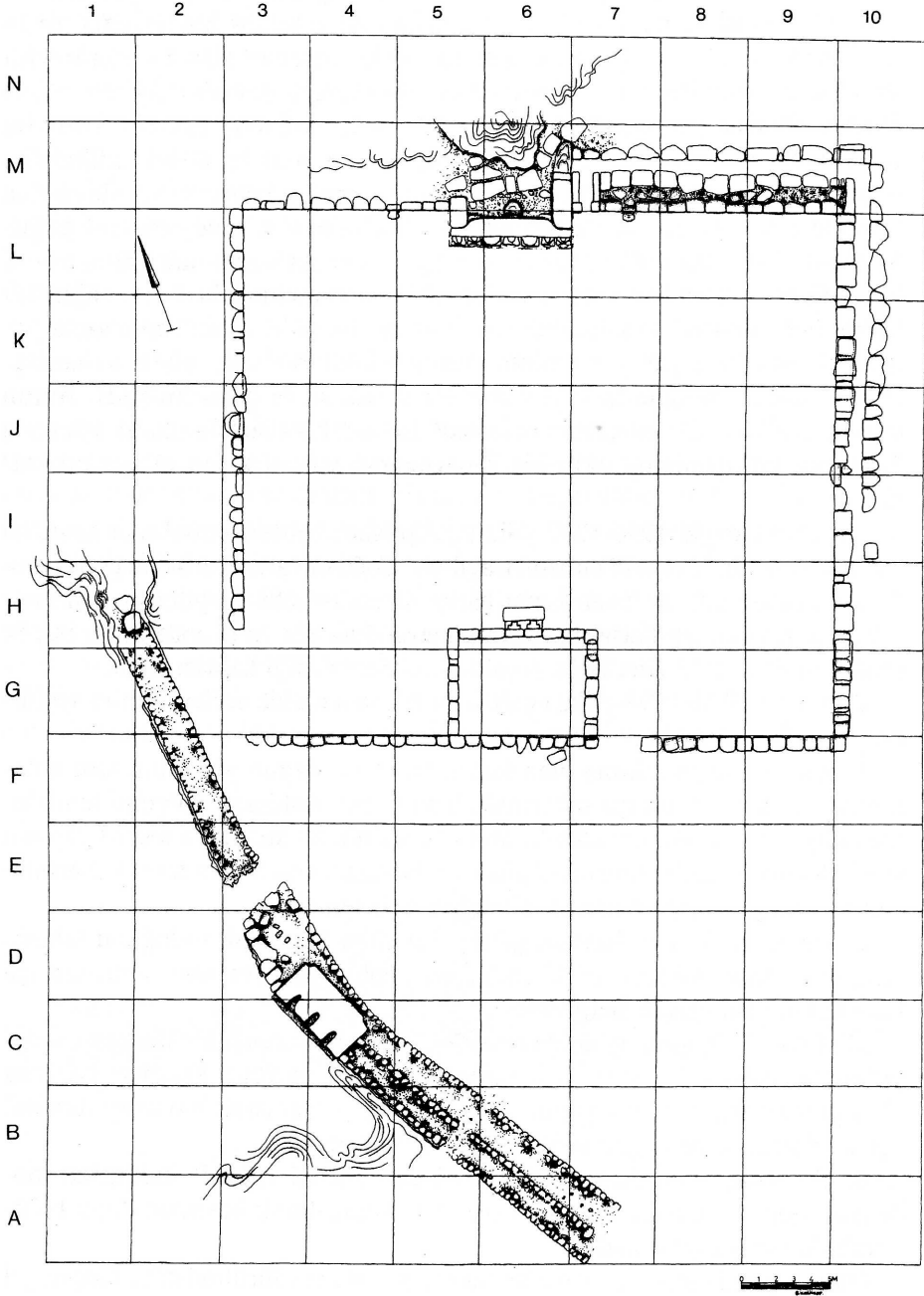
Şekil 2: Eflatunpınar Kutsal Anıt-Havuzun planı
