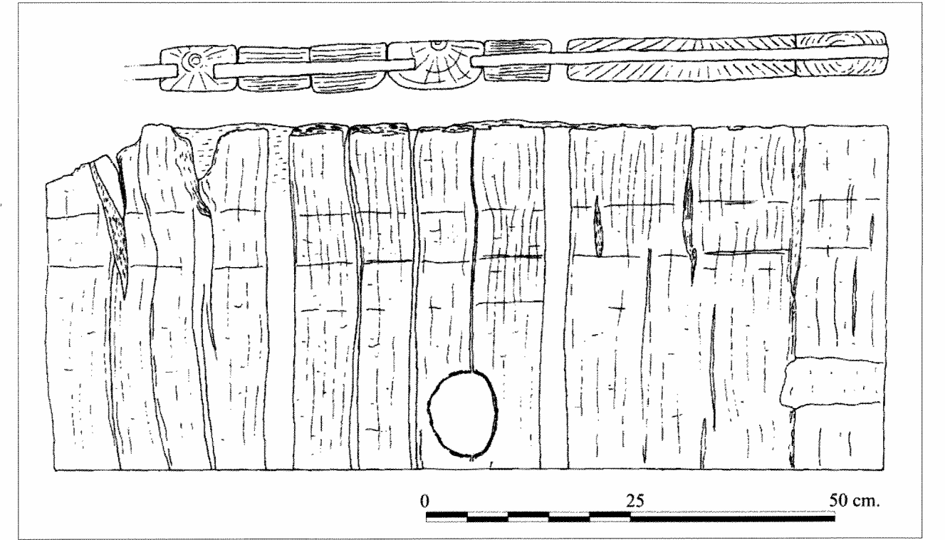
Çizim 1 Ahşap kapının sağlamlaştırılan kısmına ait detay.
